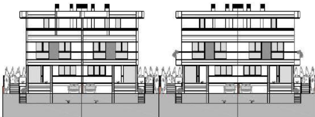
SECCIÓN ALZADO
